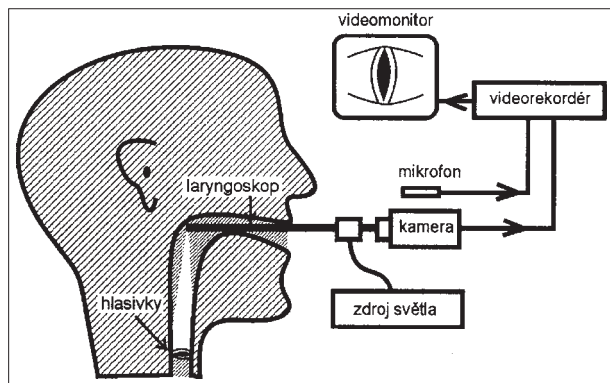
▲ Sledování hlasivek: laryngoskopické uspořádání přístrojů
