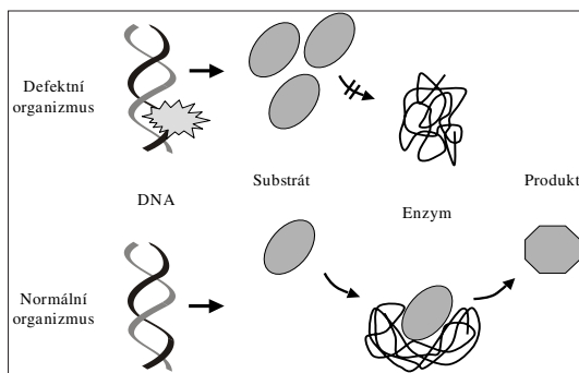
▲ Schéma zobrazující princip dědičného onemocnění metabolismu. Defektní gen v DNA produkuje protein (enzym), který není schopen uskutečnit normální konverzi substrátu na produkt. Důsledkem je hromadění substrátu a chybění produktu dané biochemické reakce
