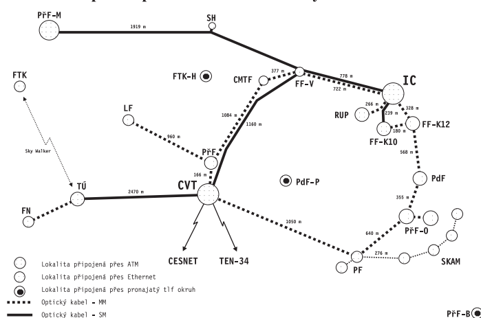
Páteř metropolitní počítačové sítě Univerzity Palackého v Olomouci.
